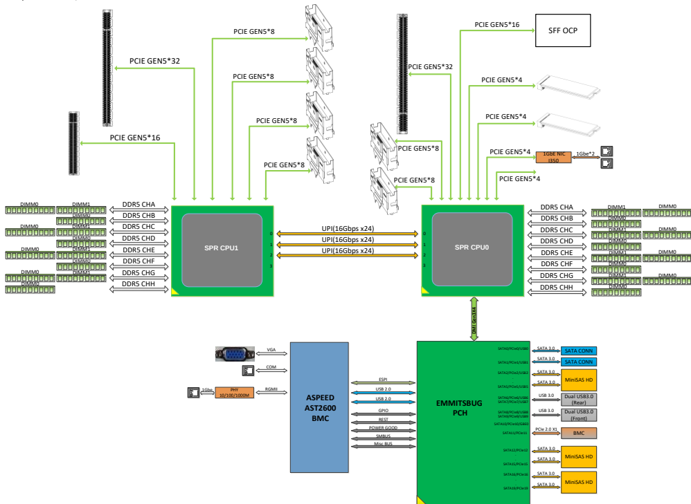
图 3.1-1 主板系统框图
