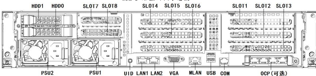
图2-9 后置面板示意图二
