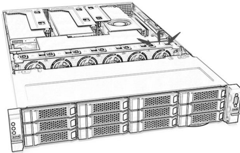
图 2-29 风扇安装与拆卸
