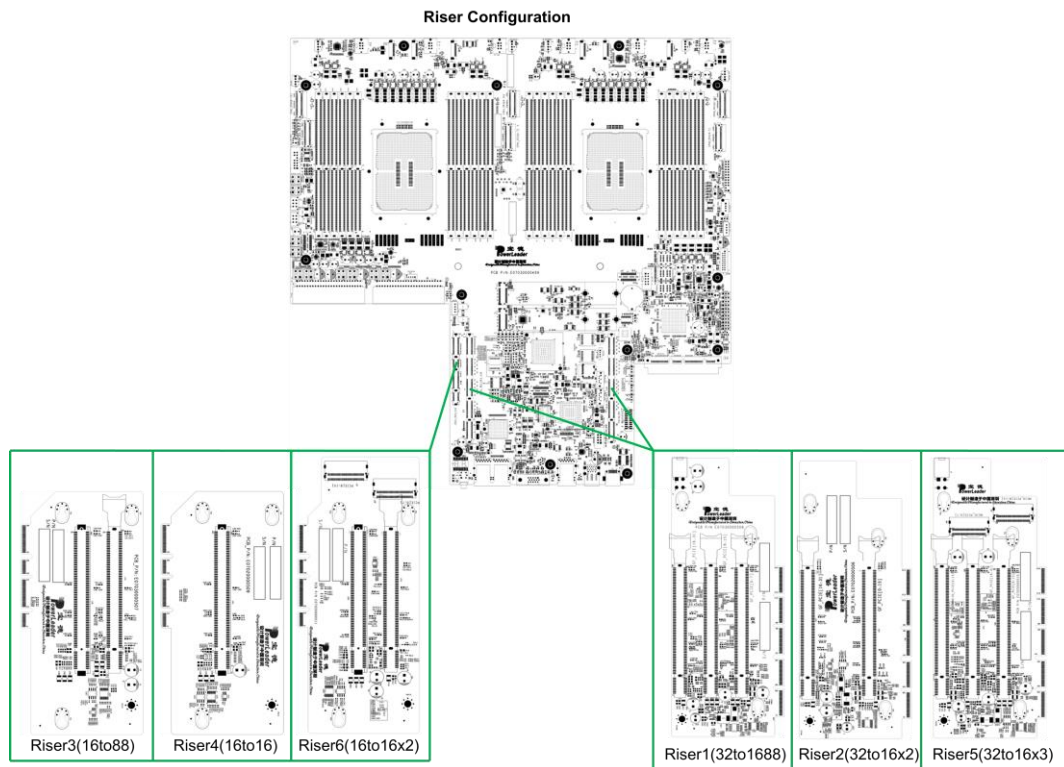
图2-11 Riser连接示意图
