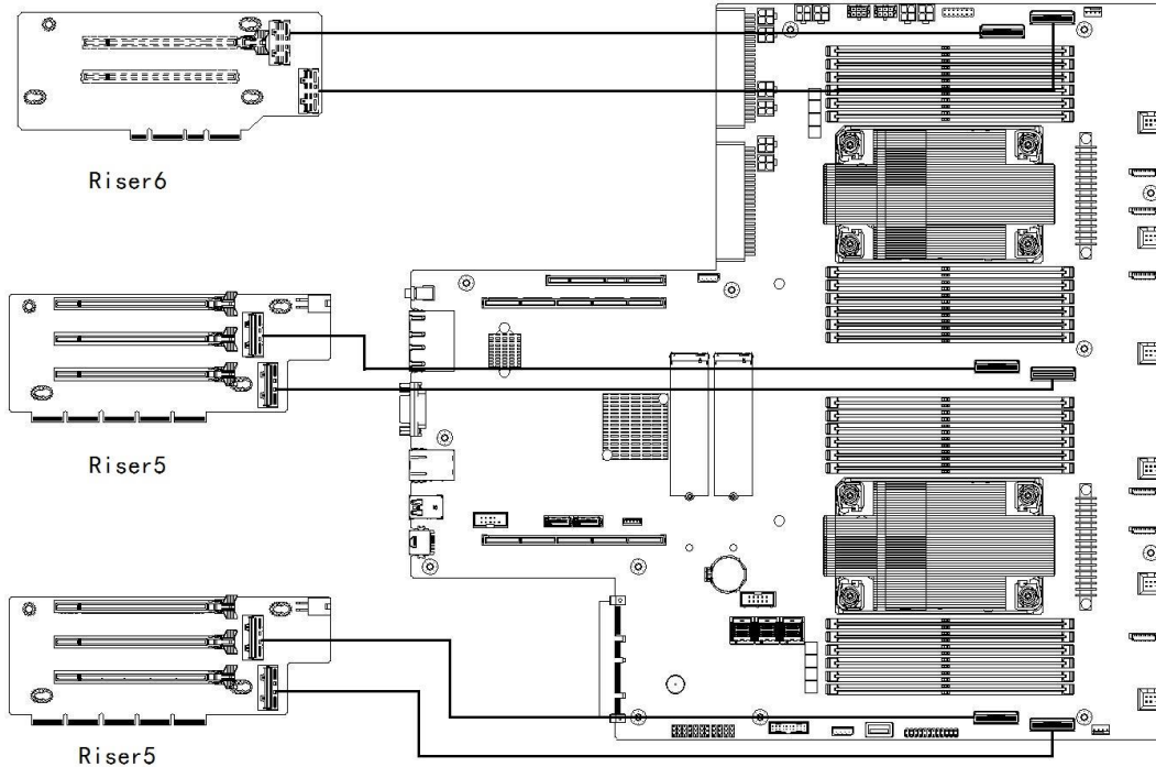
图 2-28 PCIE 转接板与主板线缆连接示意图
