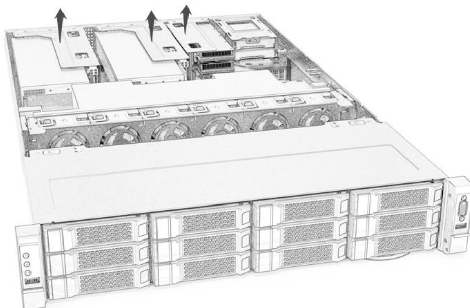
图 2-30 二个全高 PCIE 扩展模块与一个半高 PCIE 扩展模块
