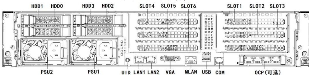
图2-10 后置面板示意图三
