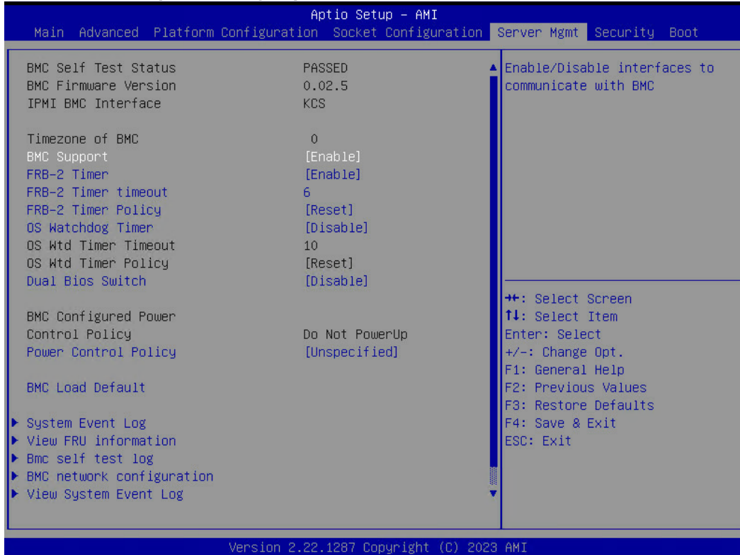
图 3.6-1 Server Mgmt 界面
