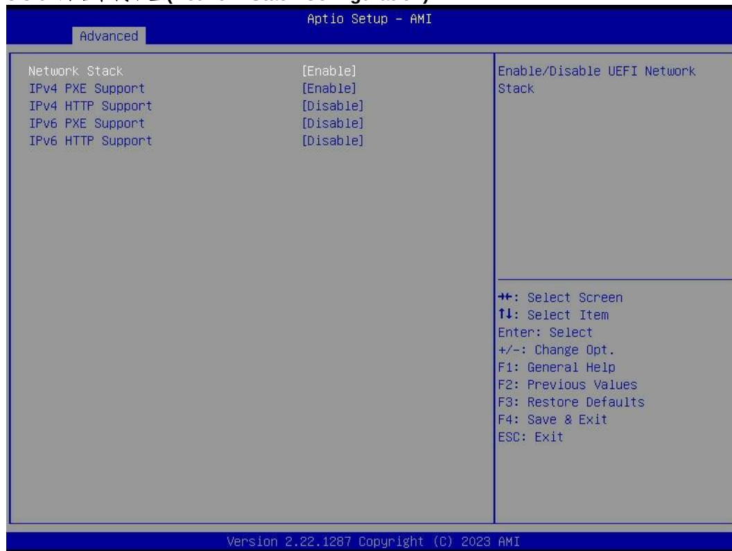
图 3.3-9 Network Stack Configuration 界面
