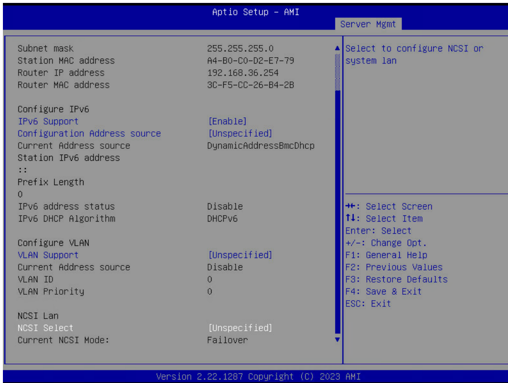
图3.6-7BMC network configuration界面
