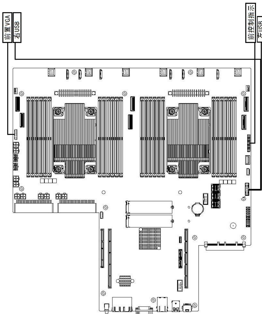
图 2-18 机箱控制面板与主板线缆连接示意图
