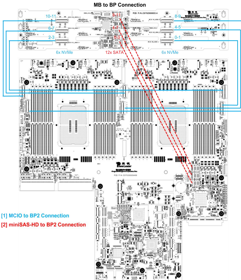
图 2-24 硬盘背板与主板线缆连接示意图二
