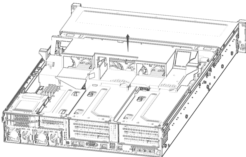
图 2-32 导风罩安装
