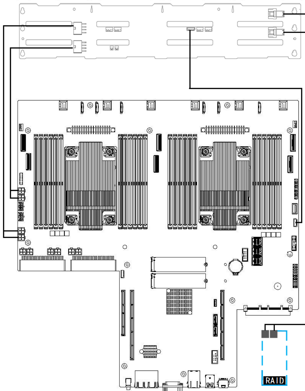
图 2-25 硬盘背板与主板线缆连接示意图三
