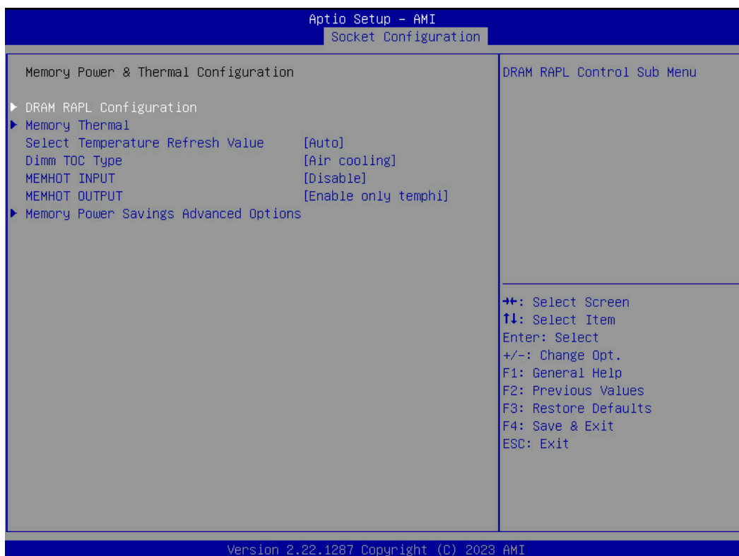
图 3.5-23Memory Power & Thermal Configuration 界面
