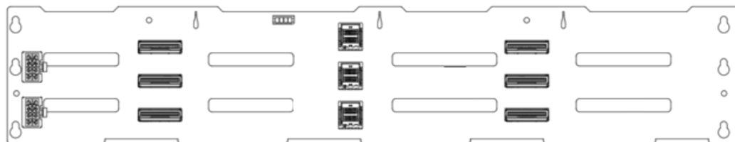
图 2-19 12 个 3.5" NVMe/SATA/SAS 硬盘背板
