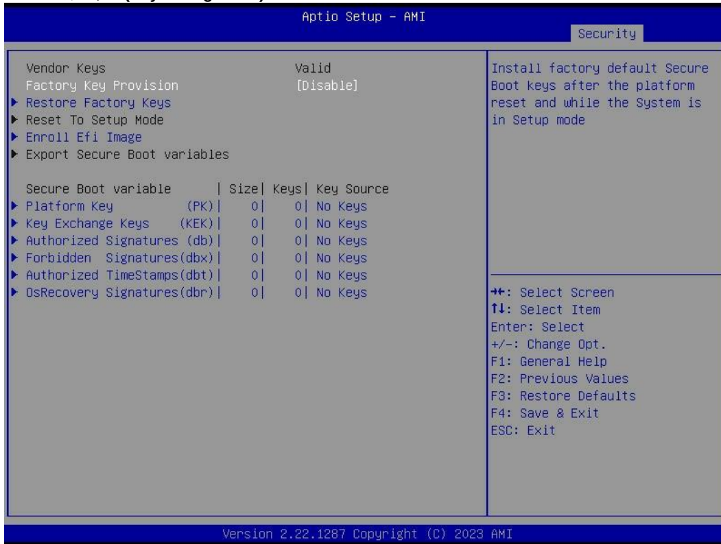
图 3.7-3 Key Management 界面
