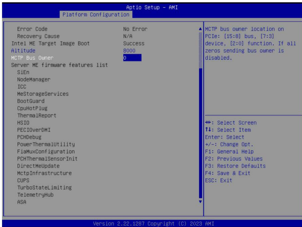
图 3.4-6 Server ME Configuration 界面
