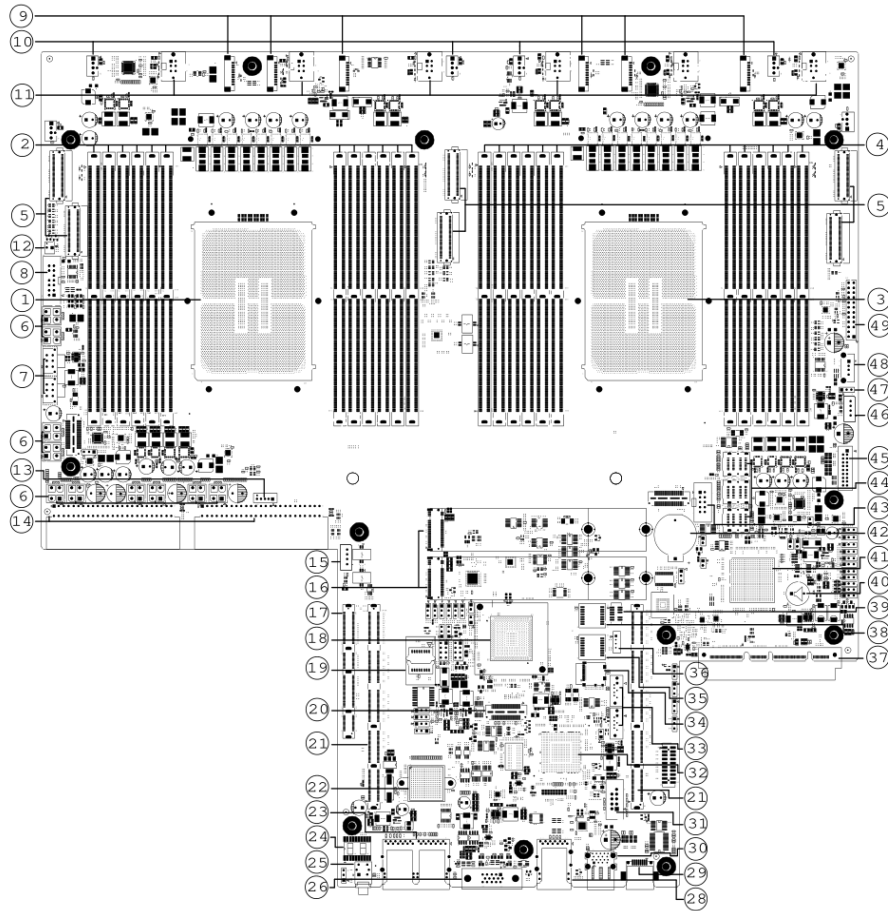
图 2-15 主板示意图
