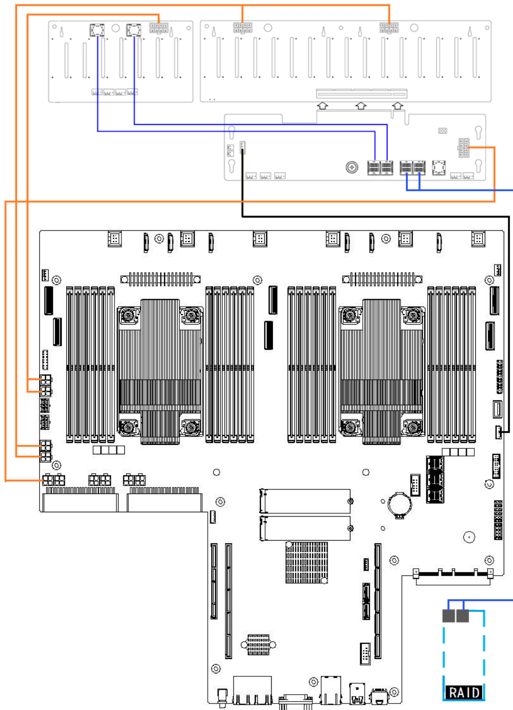
图 2-26 硬盘背板与主板线缆连接示意图四
