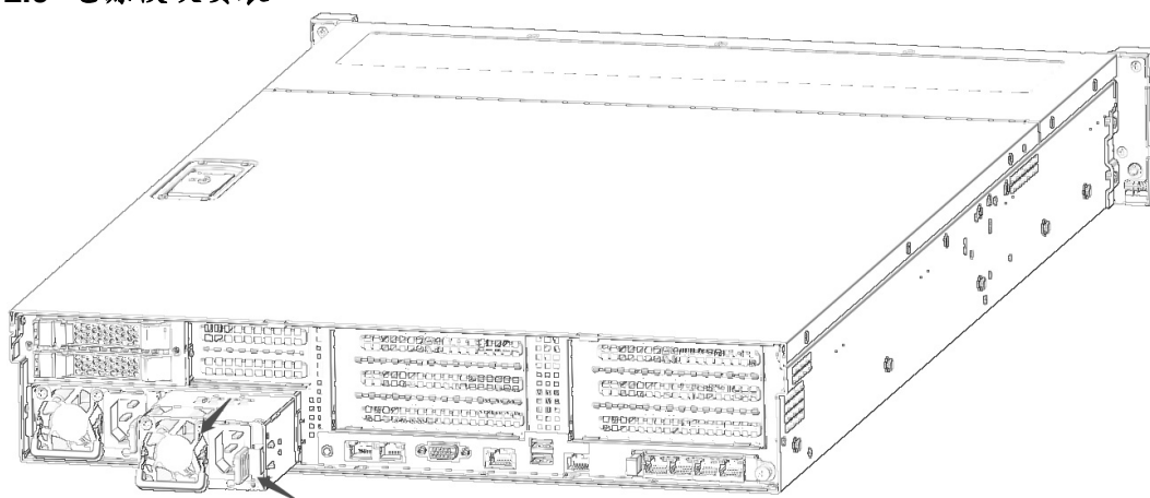
图 2-33 电源模块安装
