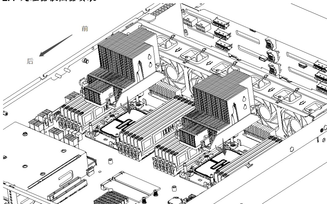
图 2-17 CPU 散热器安装位置示意图
