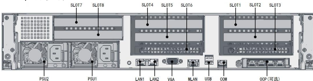
图2-8 后置面板示意图一
