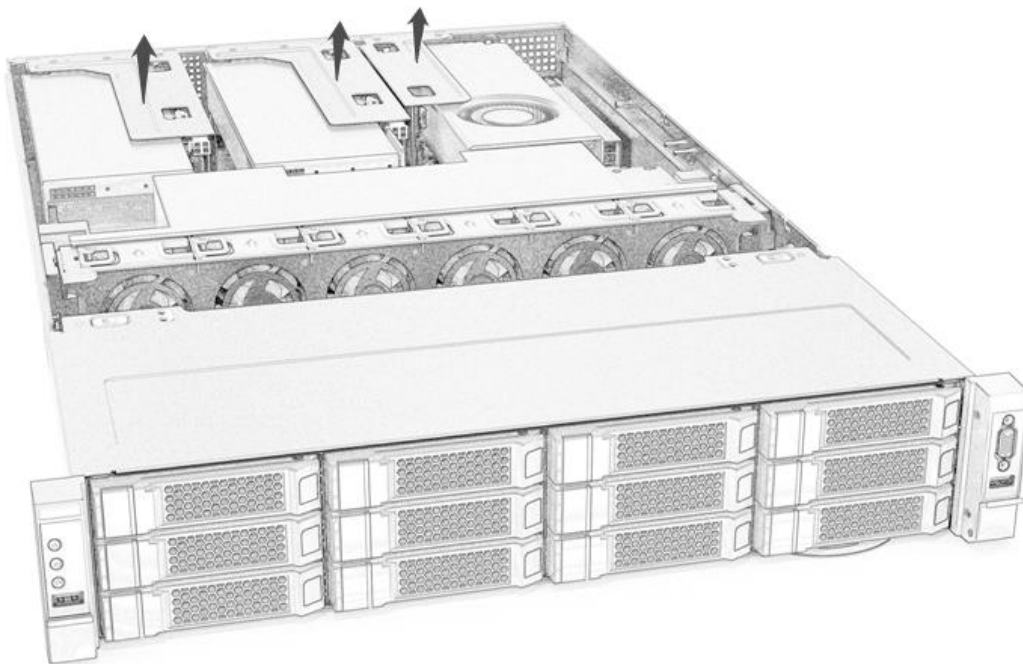
图 2-31 三个全高 PCIE 扩展模块的安装示意图
