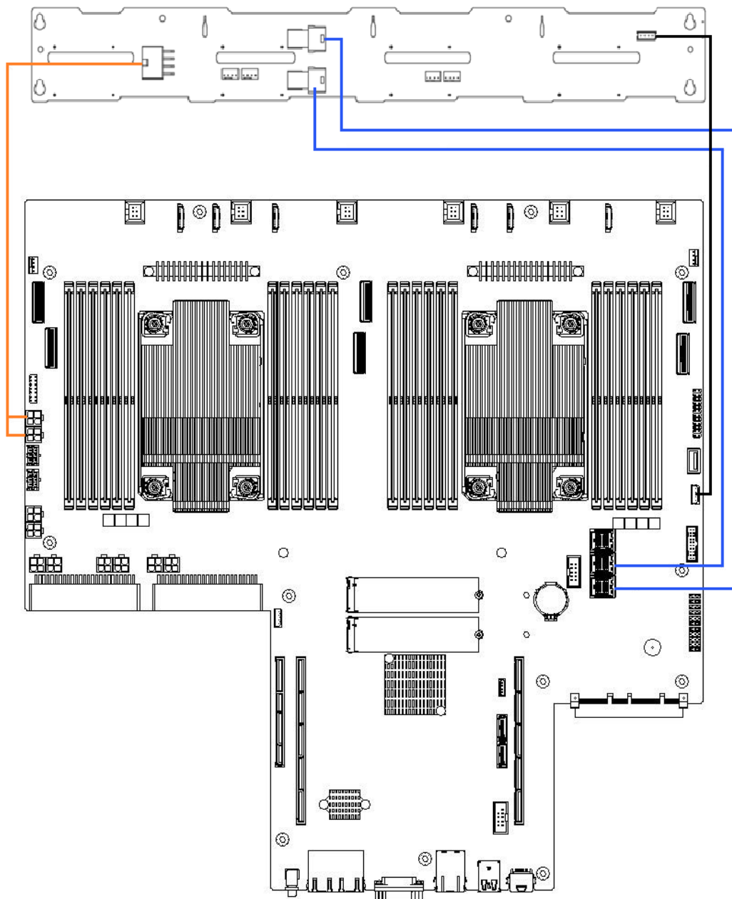
图 2-27 硬盘背板与主板线缆连接示意图五
