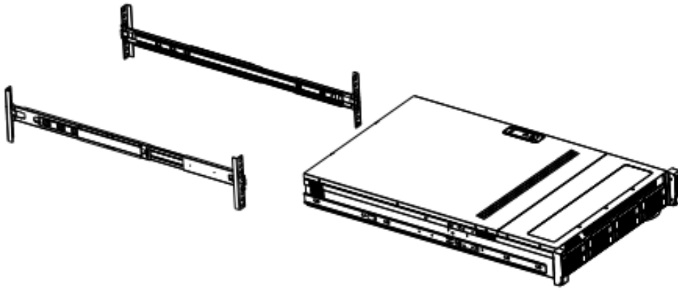
图 2-35 安装外轨
