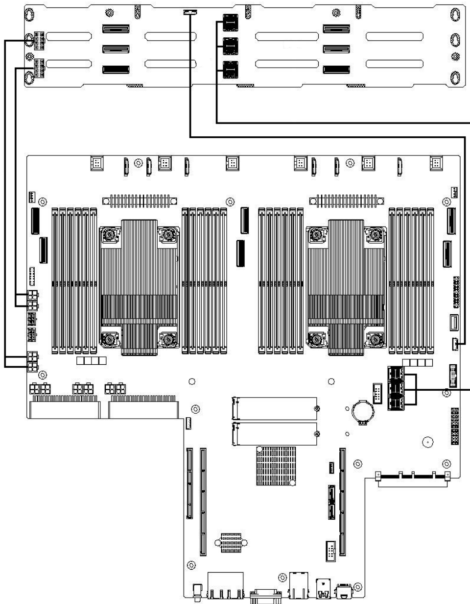
图 2-23 硬盘背板与主板线缆连接示意图一
