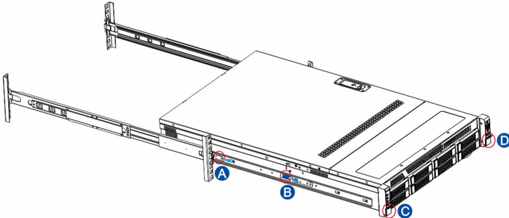
图 2-36 机箱安装到机架上
