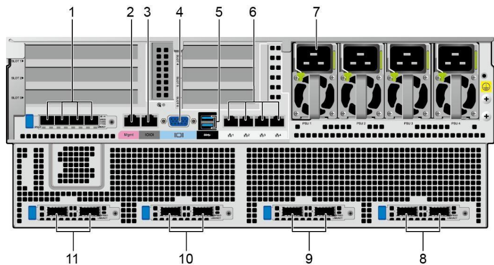
图 5-4 后面板接口示意图
