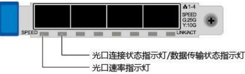
图 5-13 TM280/TM281（4*25GE/10GE 光口）
