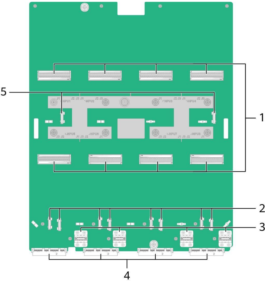
图 5-20 NPU 板接口
