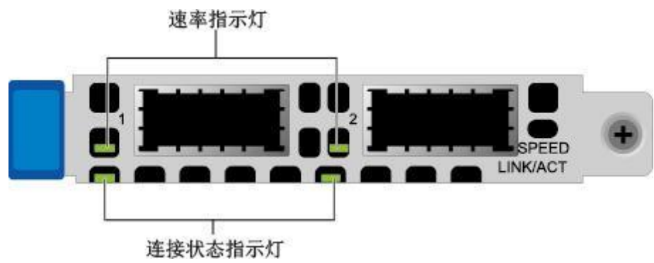
图 5-16 SF216D-H（2*200GE 光口）
