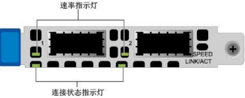
图 5-15 TM272（2*100GE 光口）
