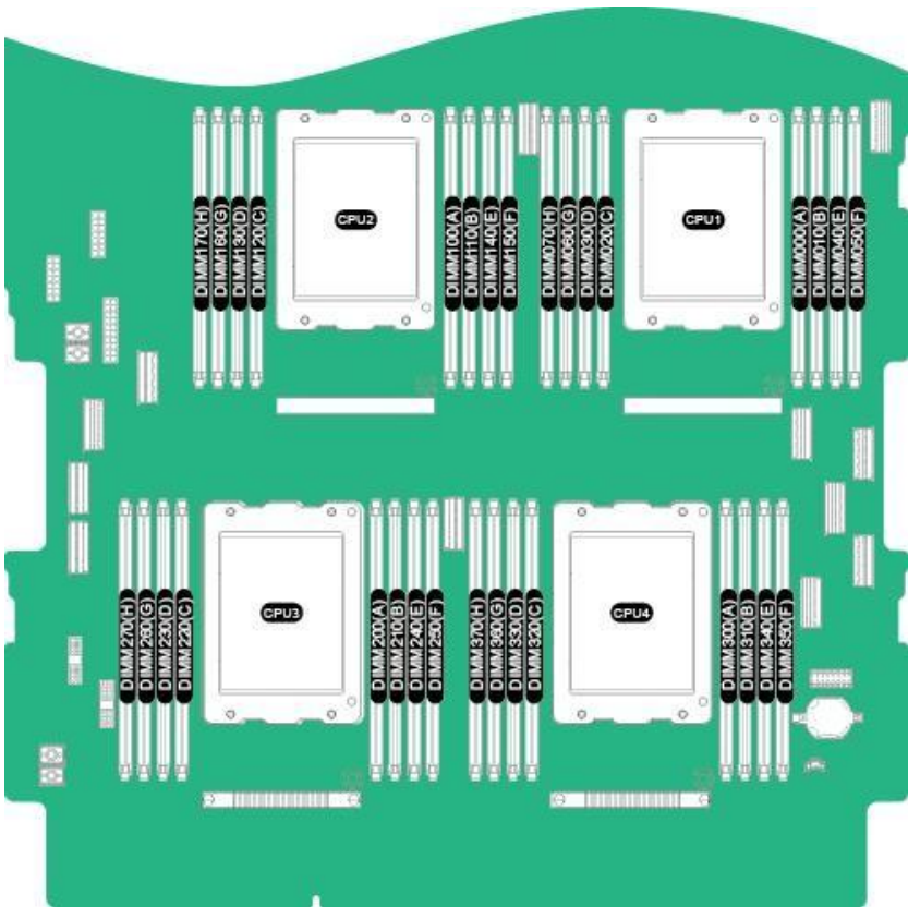
图 5-21 内存槽位编号
