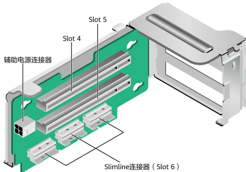
图 5-12 Riser 卡 2 示意图
