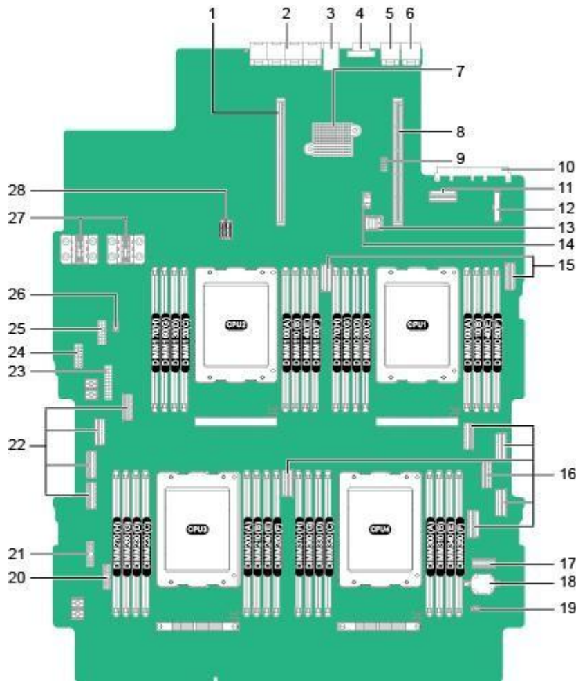
图 5-18 主板接口
