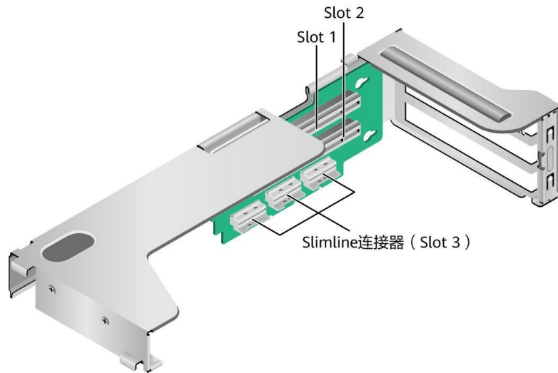
图 5-11 Riser 卡 1 示意图
