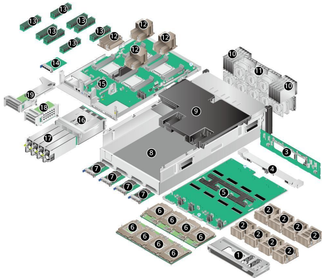
图 3-1 部件示意图
