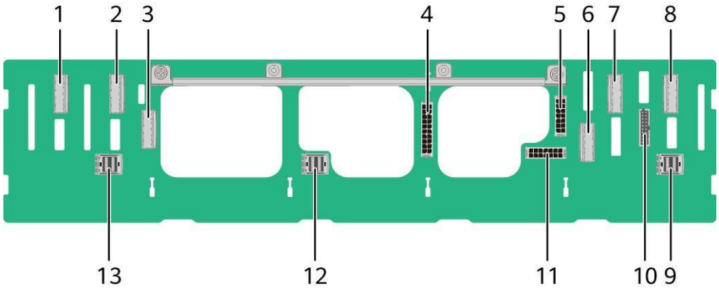
图 5-17 硬盘背板
